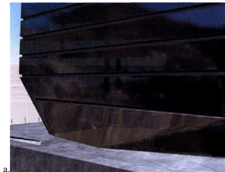
Рис. 1. Полупрозрачные детали
